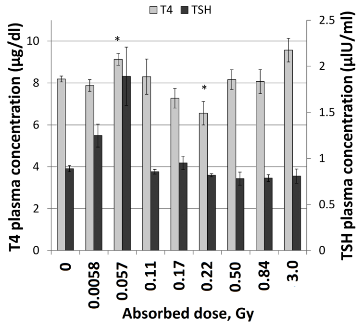
Abb. 2.3: T4 und TSH im Serum von Sprague-Dawley-Ratten als Funktion der Schilddrüsendosis 24 Stunden nach Injektion einer Salzlösung mit unterschiedlicher ^{131}\text{I} -Konzentration (aus Rudqvist et al. 2017)
