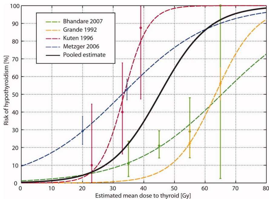
Abb. 2.2: Meta-Analyse von vier Studien des Hypothyreose-Risikos nach Strahlentherapie als Funktion der Schilddrüsendosis (aus Vogelius et al. 2011)
